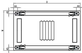
Schematic diagram of the caster bracket 防震固定示意图
